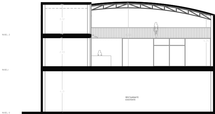
CORTE TRANSVERSAL
