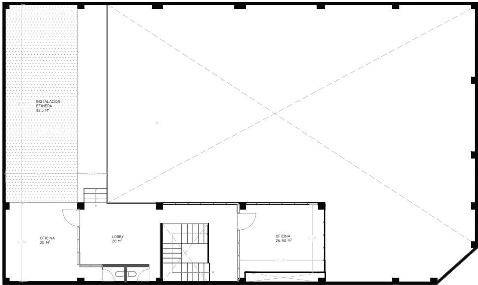
NIVEL 2
