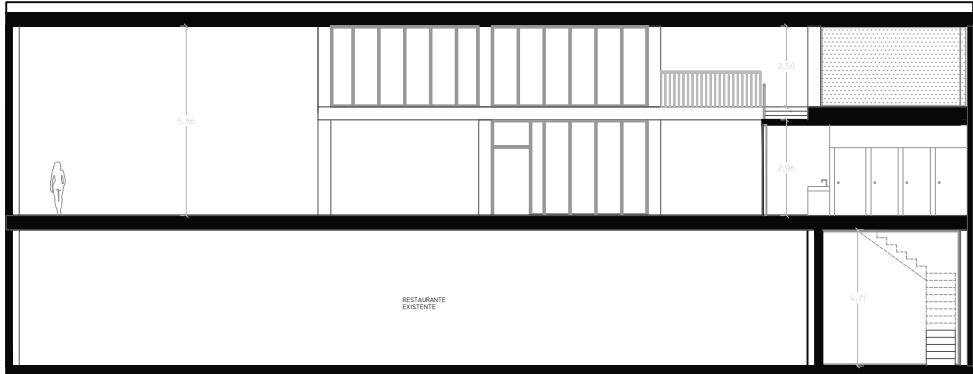
CORTE LONGITUDINAL
