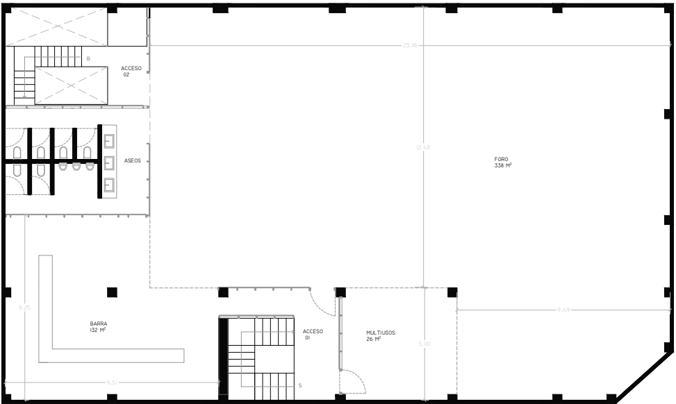
NIVEL 1
